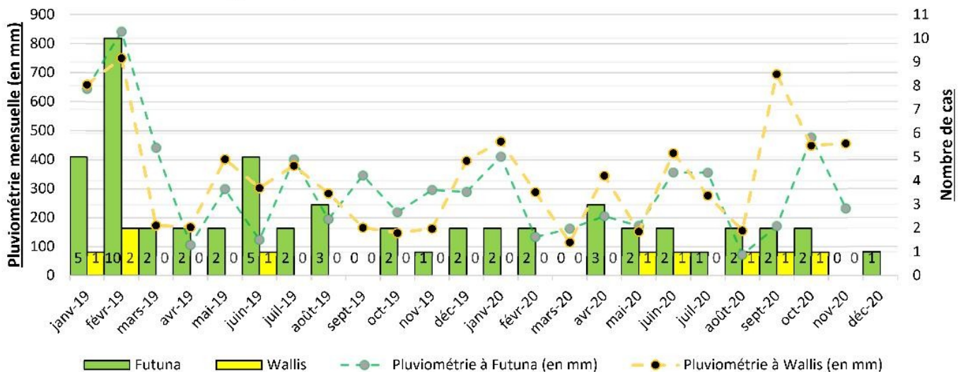
Graphique 3 : Relevé mensuel des cas de leptospirose confirmés et probables à Wallis et Futuna depuis 2019 et pluviométrie.
